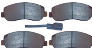
32391 410601061R JUEGO PASTILLA FRENO DELANTERA MASTER 2013>
